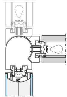
Nodo variabile da 90° a 180° Variable joint between 90° to 180° Zwischen 90° und 180° variables gelenk Angle variable de 90° à 180° Articulación variable de 90° a 180°
