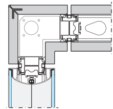
Connessione 90° modulo vetro/ modulo cieco 90° Connection glass module/ blind module 90°-Verbindung modul glas/modul blind Connections 90° module verre/ modulo plein Conexión 90° módulo vidrio/ módulo ciego
