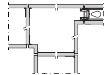
Conessioni 90°: attrezzata / div. cieca 90° Connection: equipped / blind partition 90° Verkettung: Schrankwand / Volltrennwand Connexion 90°: equipée / cloison pleine Conexión 90°: equipada / div. ciega
