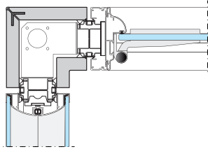
Connessione 90° modulo vetro/ porta 90° Connection glass module/ door 90°-Verbindung modul glas/modul tür Connections 90° module verre/ porte Conexión 90° módulo vidrio/ puerta
